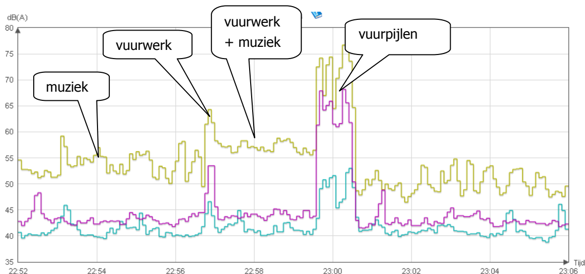
Figuur 21: overzicht gemeten geluidsniveaus rond het einde van Housequake voor locatie zuidoost (beige), villawijk (paars) en Batadorp (blauw). Het spoor is niet weergegeven omdat treinpassages het signaal sterk verstoren.
