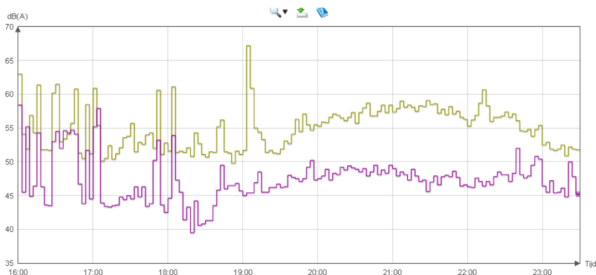
Figuur 25: overzicht gemeten geluidsniveaus rond van Frequency voor locatie zuidoost (beige) en villawijk (paars).
